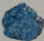
Apatite
